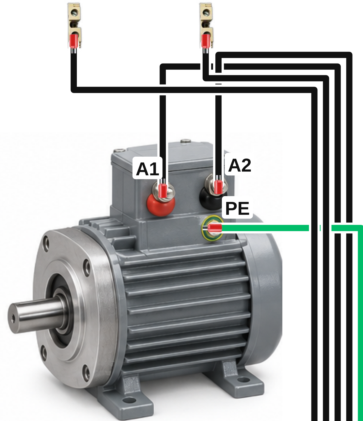
-M Motor · caixa de terminais
