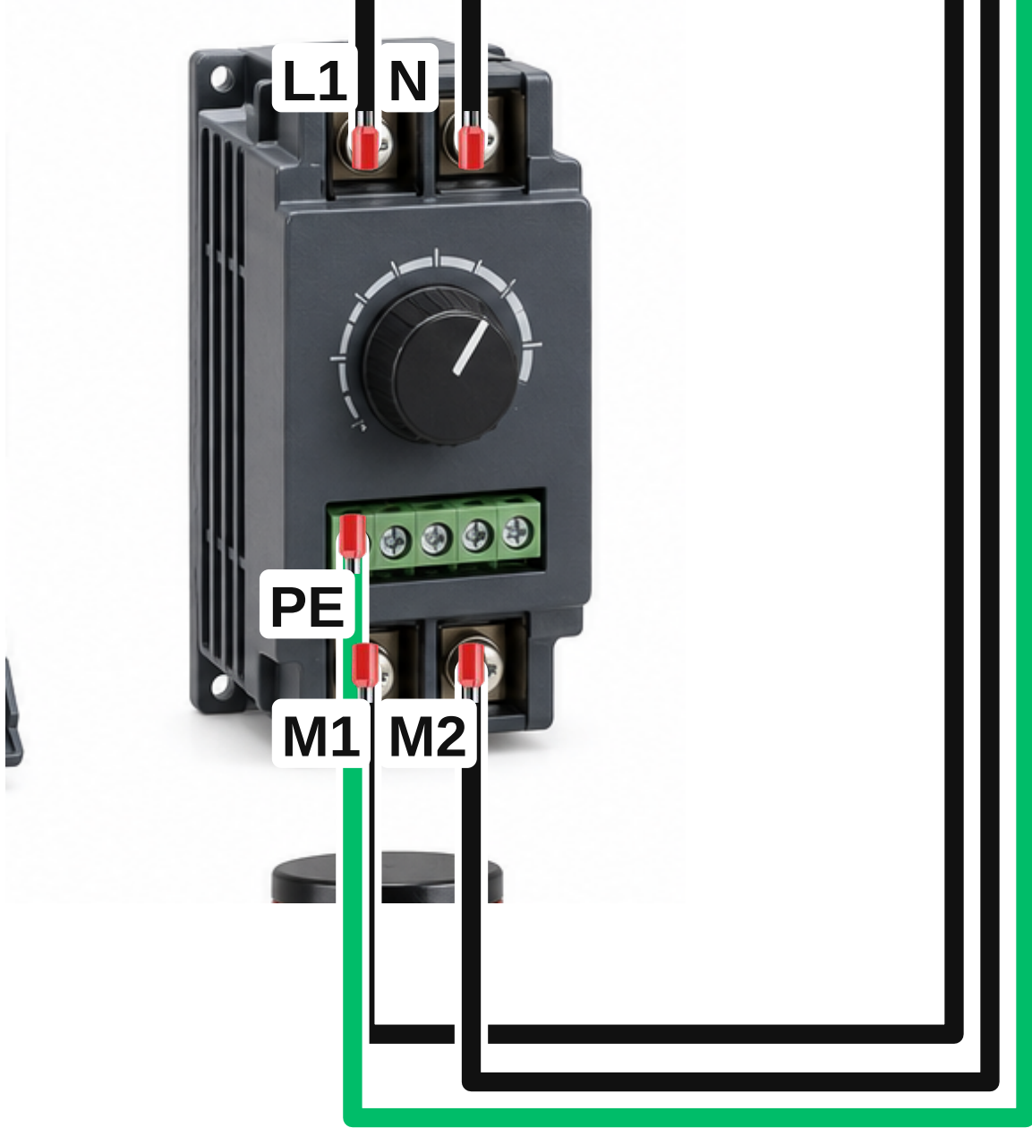
-G Conversor CC · referência
