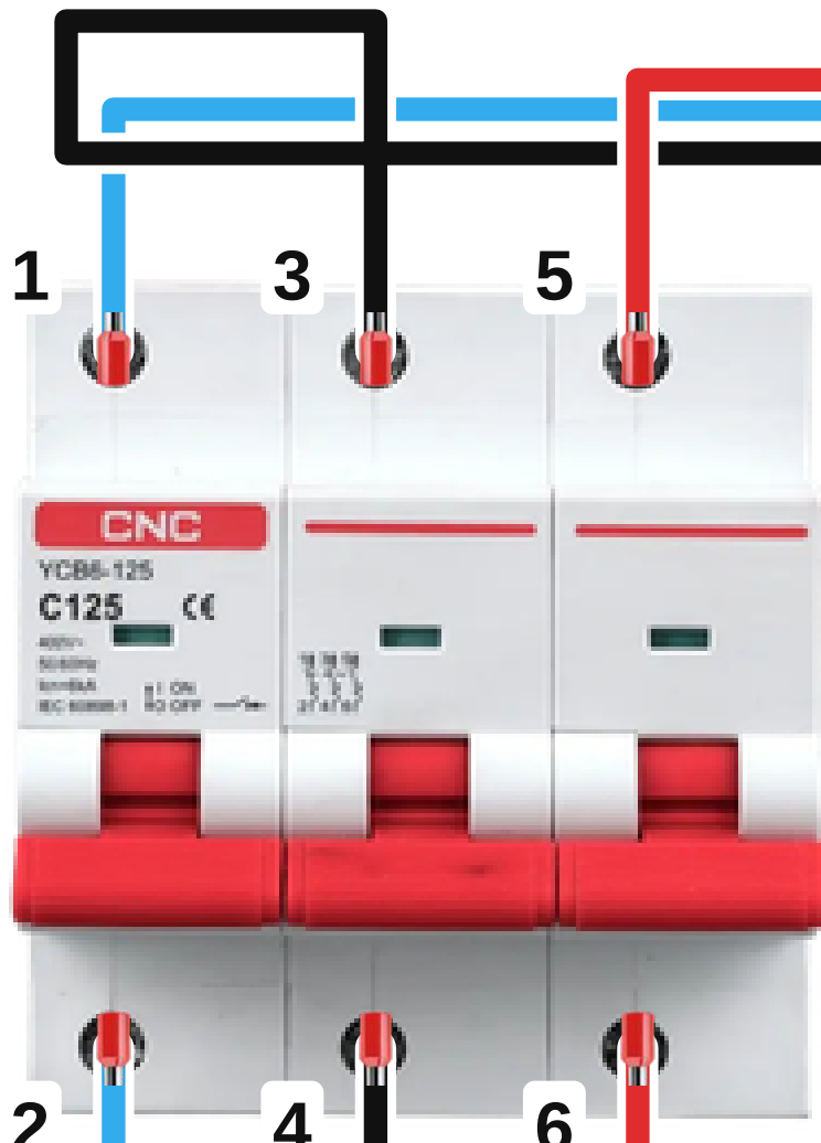
Q2 Disjuntor tripolar
